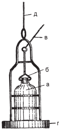
Рис. 24. Батометр: а – стерильний флакон; б – пробка; в – шнур для відкривання флакона; г – грузило; д – шнур для опускання приладу.
