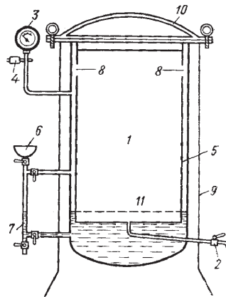
Рис. 16. Автоклав.
