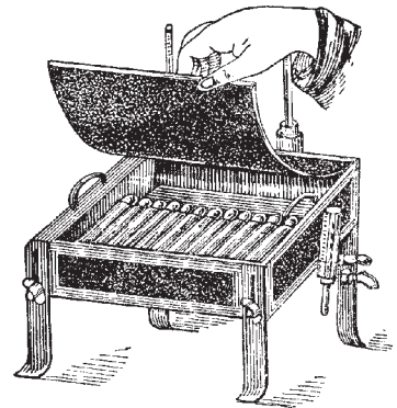
Рис. 17. Апарат для стерилізації і згортання (ущільнення) сироватки.
